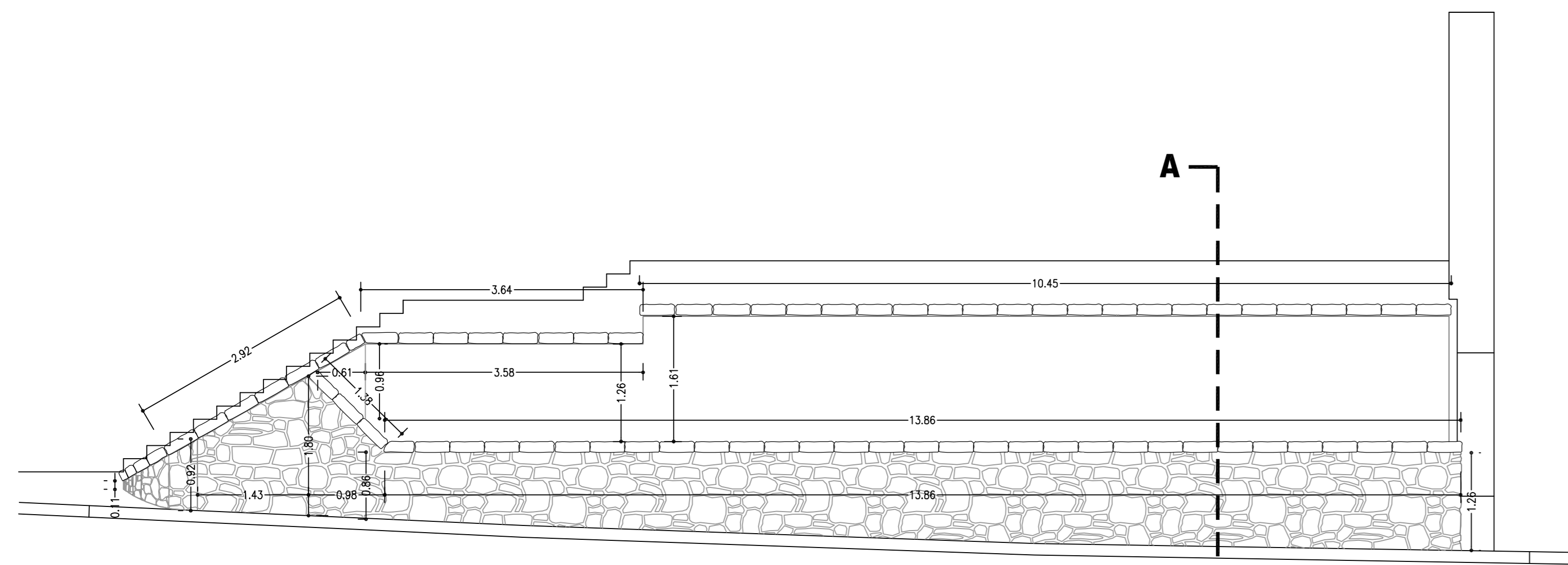
PROSPETTO MURO SCALA 1:50
